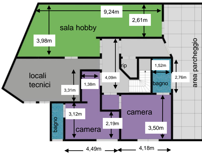
Livello inferiore h. 3,00m
